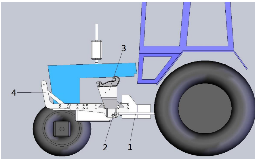
Рис.4. Навесное устройство
