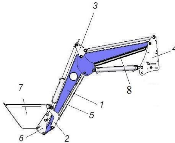
Рис.8 Подъемное устройство
