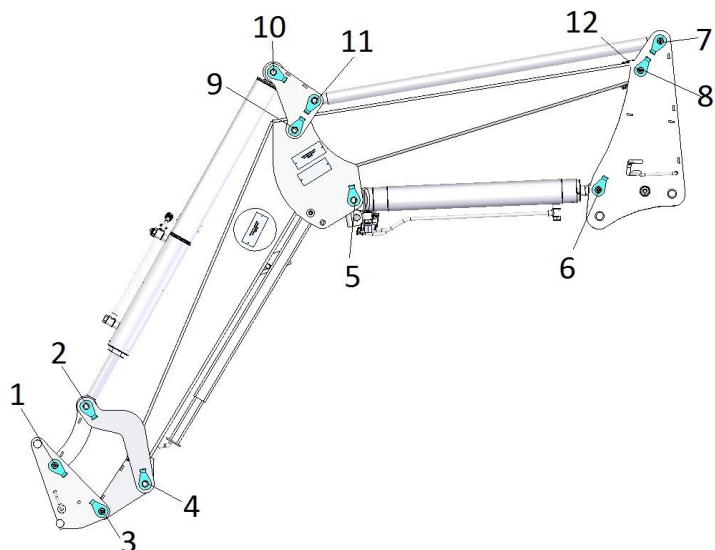
Рис.13. Схема смазки
