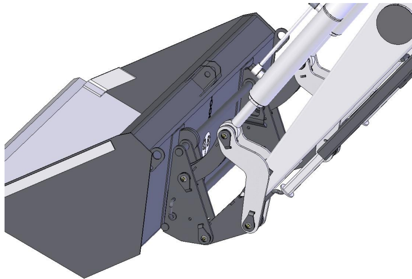
Рис.9А Установка переходника на погрузчик
